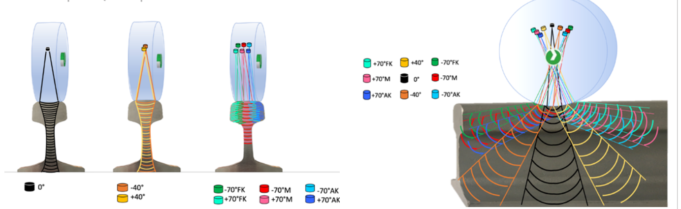
Prüfradkonzept SoniQ Rail Explorer
